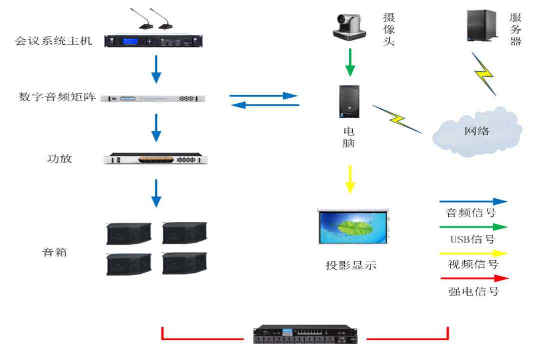
乡镇会场配置：（50 平内会议室）
