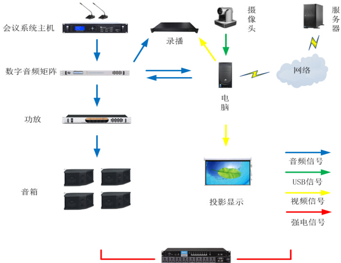
乡镇会场配置：（50 平内会议室）
